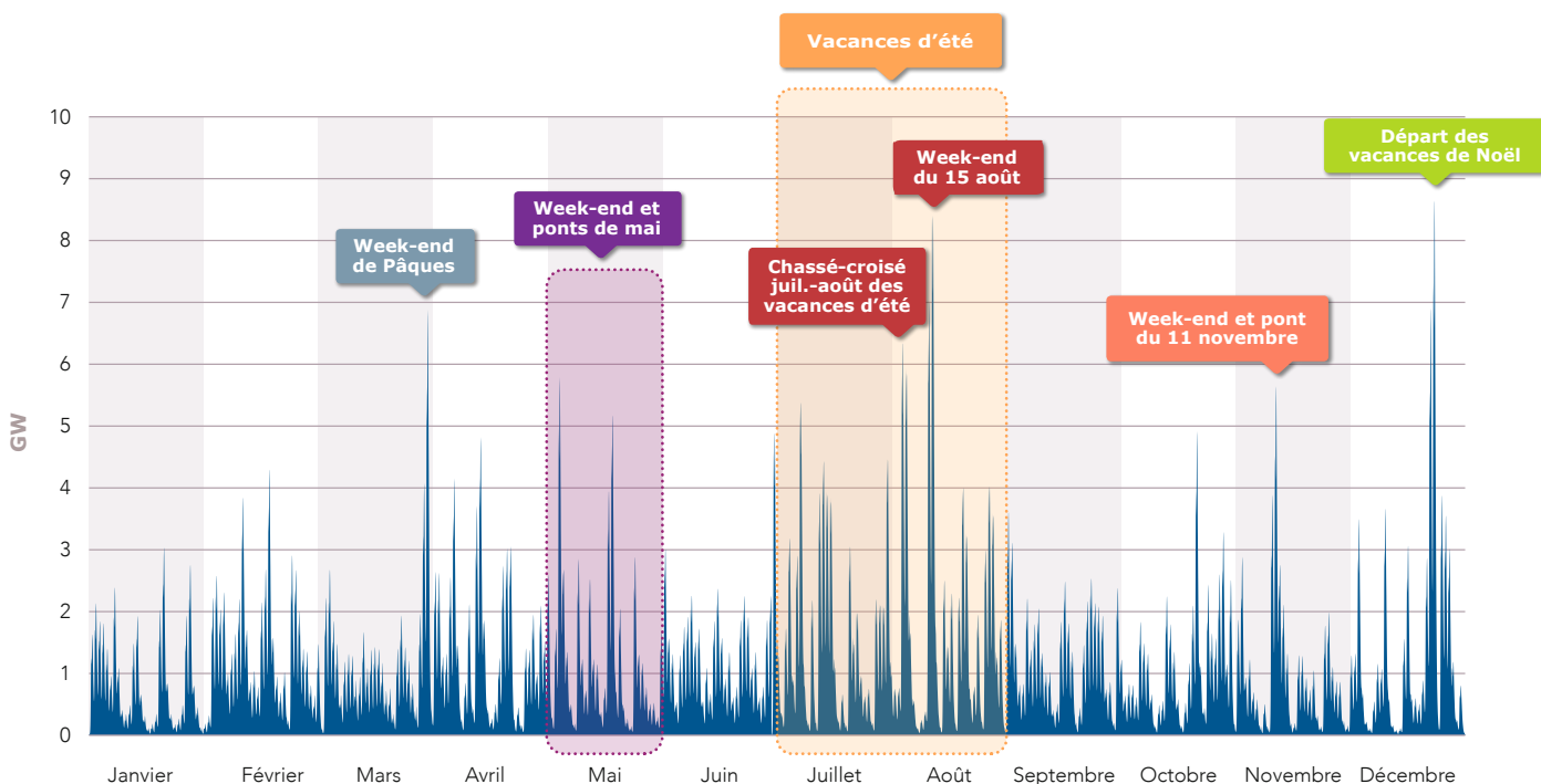
Figure 9. Puissance soutirée pour les besoins de mobilité longue distance dans le scénario Forte haut (cumul de la puissance soutirée en itinérance sur les axes routiers et de la puissance soutirée à destination).
