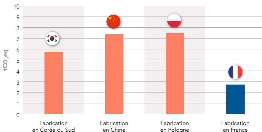
Figure 33. Analyse de cycle de vie d'une batterie de 40 kWh à l'heure actuelle selon le lieu de fabrication (hors prise en compte du recyclage)
